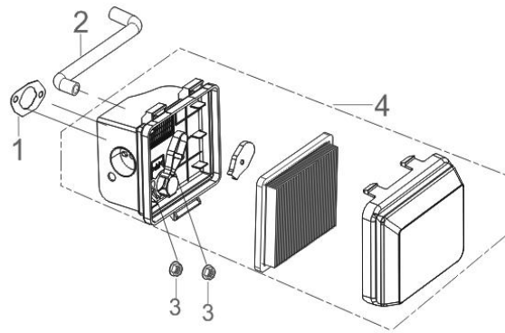
FIG.9 CLEANER, AIR 空滤器 ( E09 )
